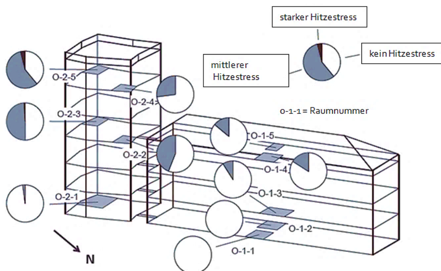
Abbildung 51: Verteilung des Hitzestresses in zwei Berliner Nichtwohn-Gebäuden in den Sommermonaten 2011/ 2012. Quelle: LANGNER et al. 2014: 267 (Eigene Übersetzung).
