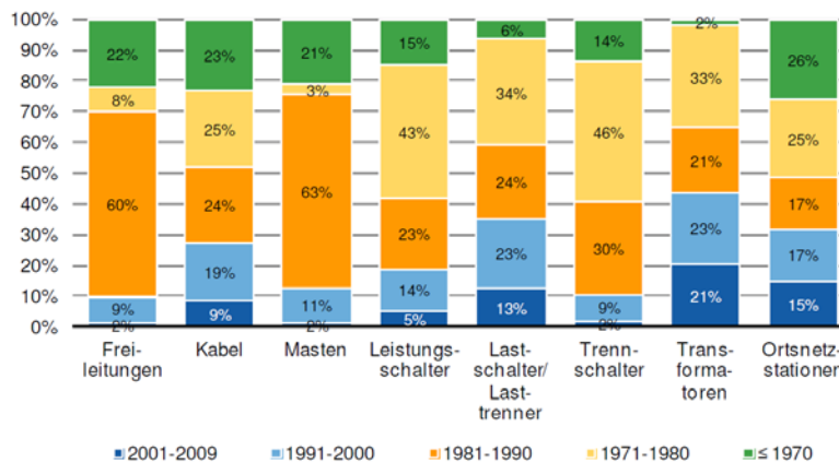
Abbildung 71: Jahr der Inbetriebnahme verschiedener Bestandteile des Berliner Stromnetzes (Stand: 2010). Quelle: VATTENFALL 2011.
