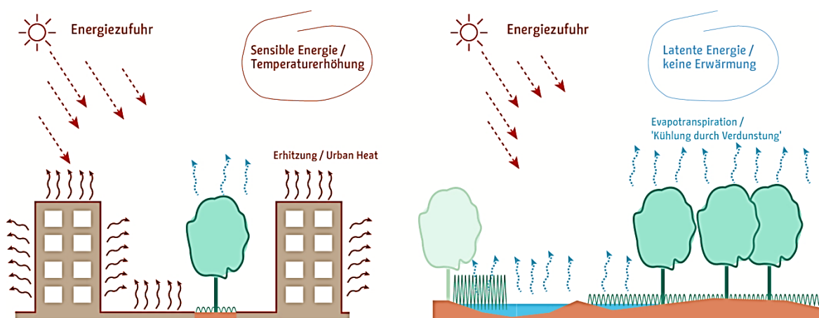
Abbildung 44: Veränderung der klimatischen Situation bei unterschiedlicher Verdunstungskapazität von Oberflächen führt zu sensibler (links) und latenter (rechts) Energie. Quelle: BBSR 2015b: 38; Grafik BGMR LANDSCHAFTSARCHITEKTEN, verändert.
