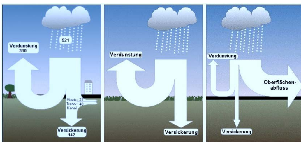
Abbildung 56: Links: Gesamtwasserhaushalt Berlins; langjährige Mittelwerte in Mio. m 3 ohne Gewässer 66 ; Mitte: Wasserhaushalt Vegetationsfläche; rechts: Wasserhaushalt versiegelte Fläche. 67
