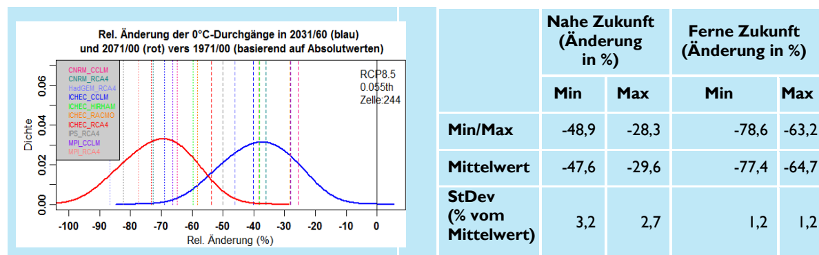
Abbildung 14: Relative Änderung der Variable „Glatteistage“ für Berlin (Gitterzelle Dahlem) – Zeitreihen der CORDEX-Modellergebnisse (links) und die über alle betrachtete Gitterzellen aggregierte Änderung der Mehrheit der Modelle (Tabelle rechts). Quellen: Eigene Berechnungen – siehe Text.
