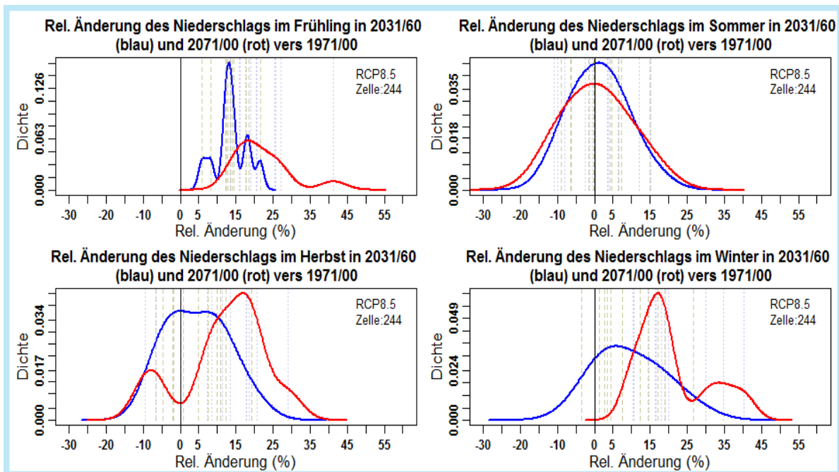
Abbildung 16: Jahreszeitliche Betrachtung der relativen Änderungen in der Niederschlagssumme in der Gitterzelle Dahlem. Quellen: Eigene Berechnungen – siehe Text.
