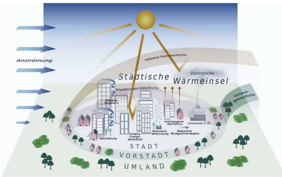
Abbildung 43: Schematische Darstellung der städtischen Wärmeinsel. Quelle: DEUTSCHER WETTERDIENST. 58
