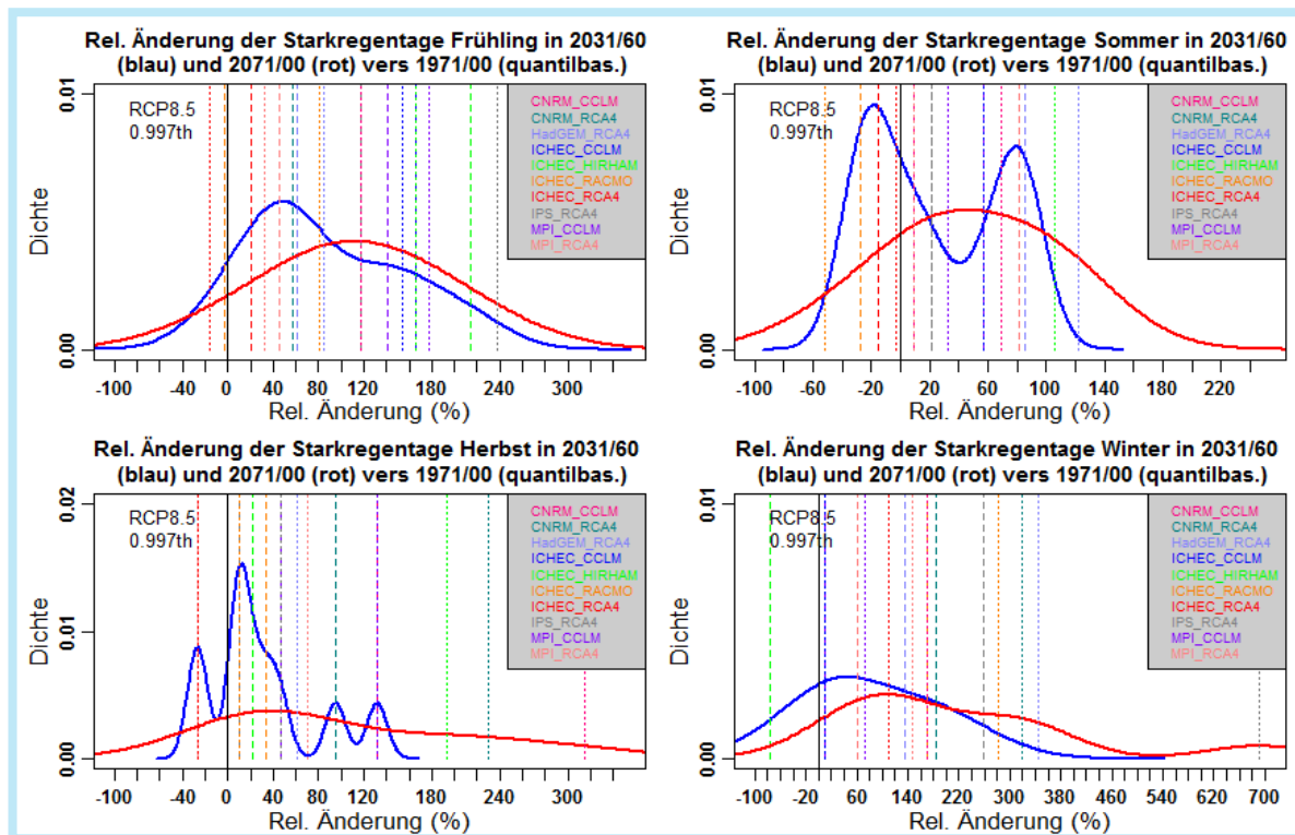
Abbildung 19: Jahreszeitliche Betrachtung der relativen Änderungen der Starkniederschlagstage in der Gitterzelle Dahlem. Quelle: Eigene Berechnungen – siehe Text.
