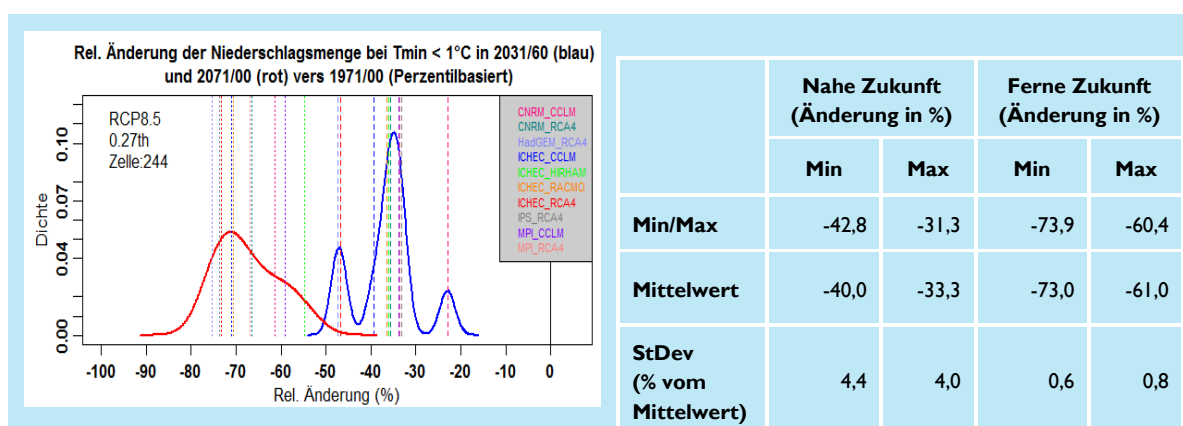
Abbildung 20: Relative Änderung der Variable „Niederschlag an Tagen unter 1°C“ für Berlin (Gitterzelle Dahlem) – Verteilung der Häufigkeitsänderungen (links) und die über alle betrachteten Gitterzellen aggregierte Änderung der Mehrheit der Modelle (Tabelle rechts). Quellen: Eigene Berechnungen – siehe Text.
