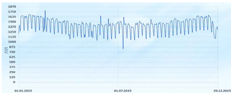
Abbildung 66: Lastgang im Berliner Stromnetz vom 1.1. bis 31.12.2015. Quelle: STROMNETZ BERLIN GMBH o.J.
