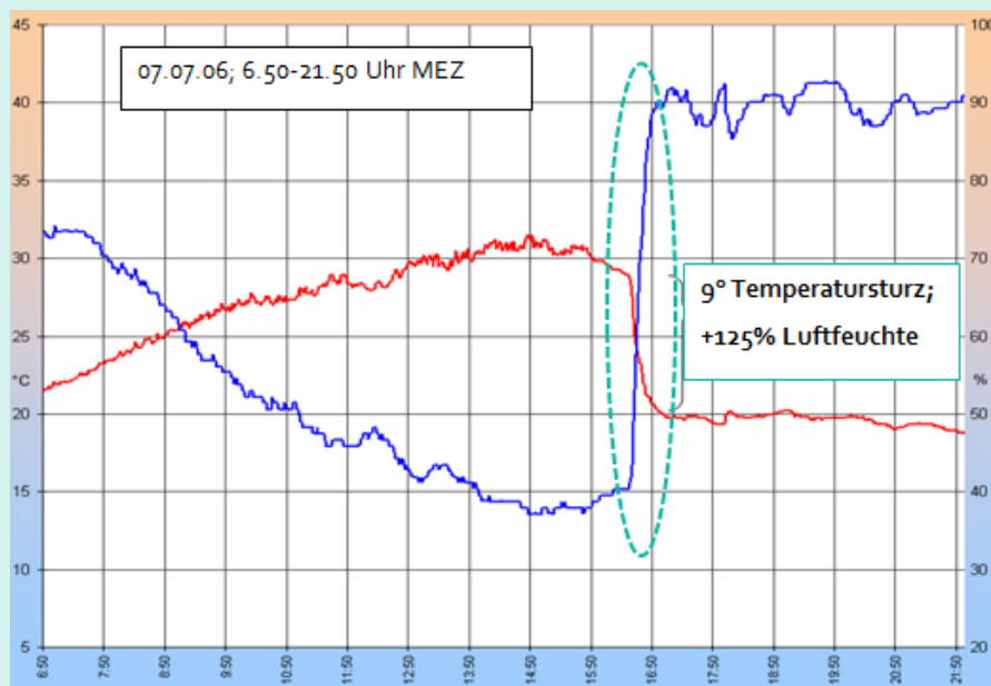
Abbildung 34: Abrupte Entwicklung (grün gestrichelter Bereich umfasst ca. 1 Stunde) von Temperatur (rot) und starkregenbedingter Schwankung der Luftfeuchte (blau) (Station der FU im Botanischen Garten, Dahlem) am 07.07.2006. Quelle: JANKIEWICZ/ MYRCIK/ WEHRY 2006: 4.
