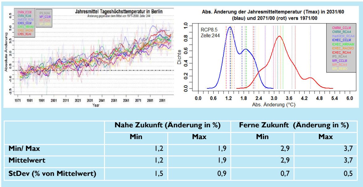
Abbildung 9: Änderung der Variable „Tageshöchsttemperatur“ für Berlin (Gitterzelle Dahlem) – Zeitreihen der CORDEX-Modellergebnisse (oben links), Verteilung der absoluten Temperaturänderungen (oben rechts) und die über alle betrachtete Gitterzellen aggregierte Änderung der Mehrheit der Modelle 18 ; (Tabelle unten). Quellen: Eigene Berechnungen – Siehe Text.
