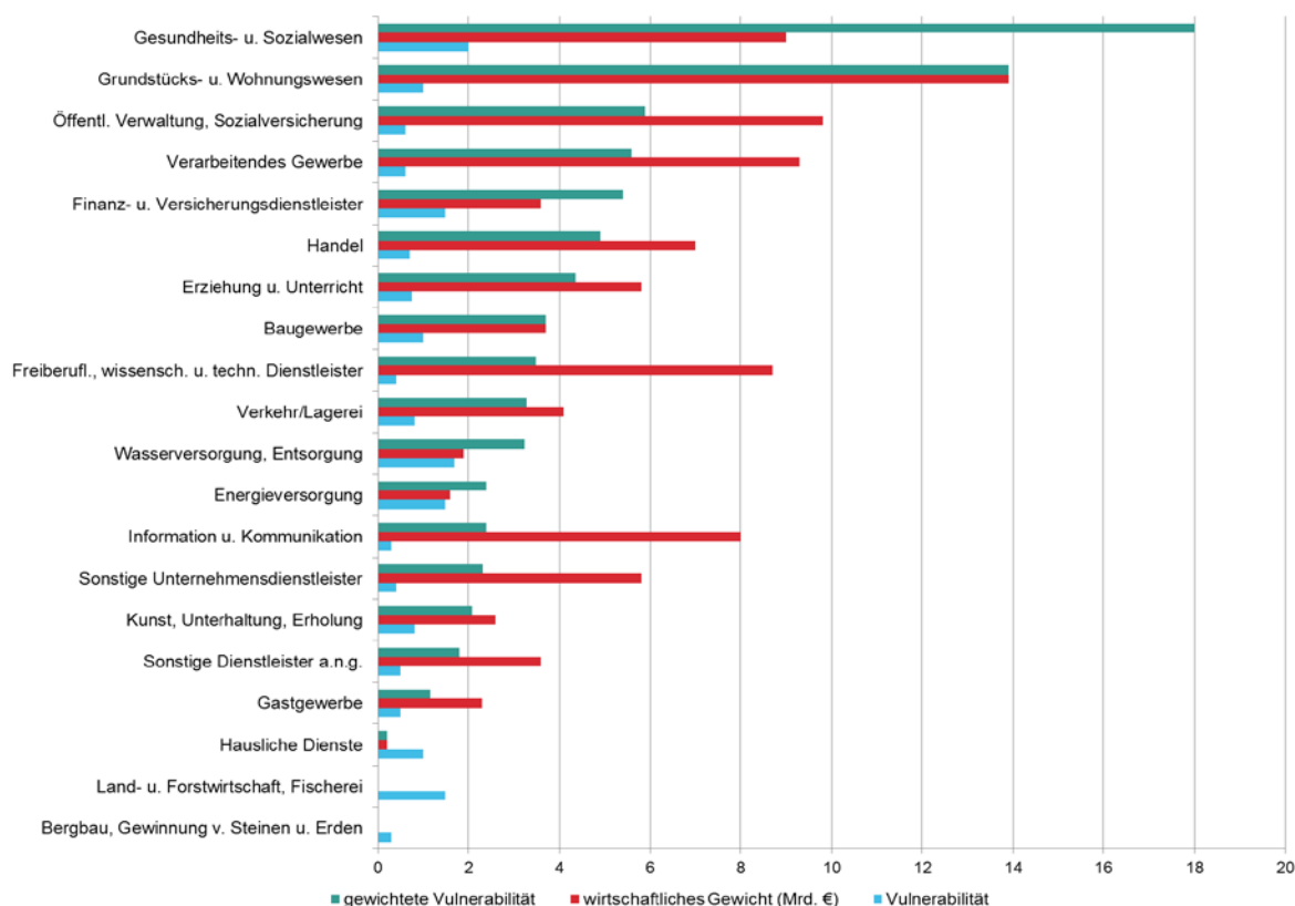
Abbildung 76: Vulnerabilität (blau), wirtschaftliches Gewicht (rot) und gewichtete Vulnerabilität (grün) der Berliner Wirtschaft nach Wirtschaftsbereichen. Quelle: Eigene Darstellung.
