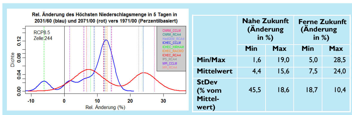
Abbildung 17: Relative Änderung der Variable „Höchste Niederschlagsmenge in 5 Tagen“ für Berlin (Gitterzelle Dahlem) - Verteilung der Häufigkeitsänderungen (links) und die über alle betrachtete Gitterzellen aggregierte Änderung der Mehrheit der Modelle (Tabelle rechts). Quellen: Eigene Berechnung – siehe Text.
