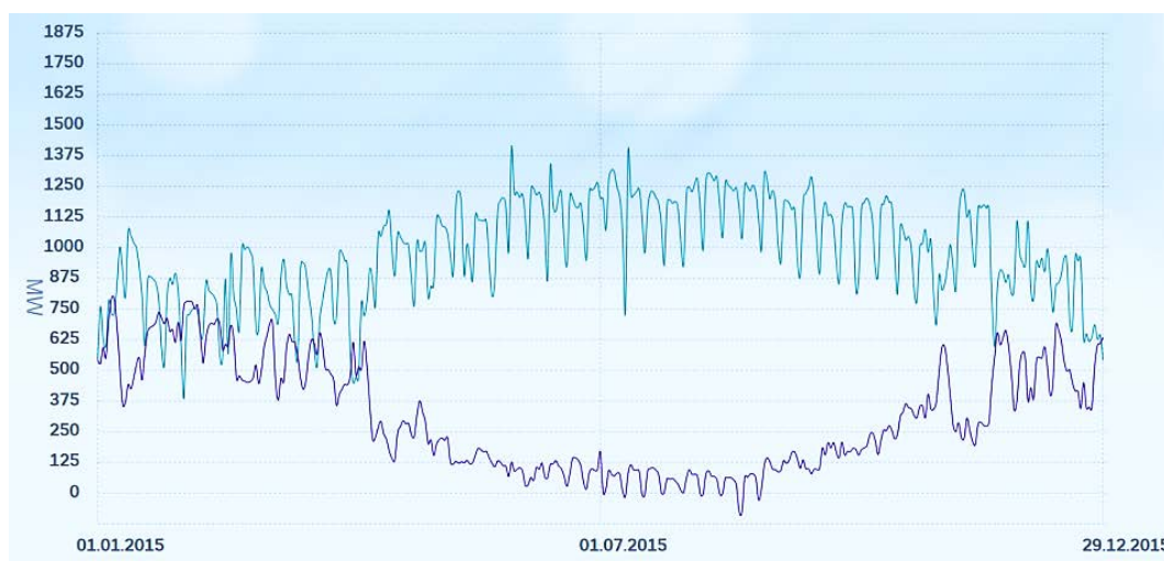
Abbildung 68: Eigenerzeugung (violette Linie, unten) und Stromimporte (grüne Linie, oben) im Last-gangprofil des Jahres 2015. Quelle: STROMNETZ BERLIN GMBH O.J.
