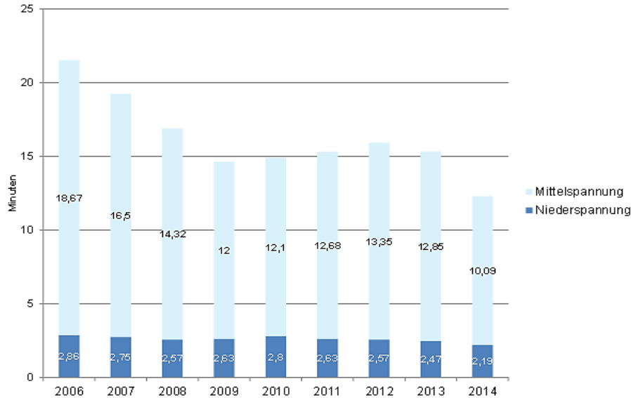
Abbildung 70: Dauer der Versorgungsunterbrechungen (SAIDI) im deutschen Stromnetz (hellblau: Mittelspannung, dunkelblau: Niederspannung) in Minuten. Quelle: Eigene Darstellung auf Basis von Daten der Bundesnetzagentur.
