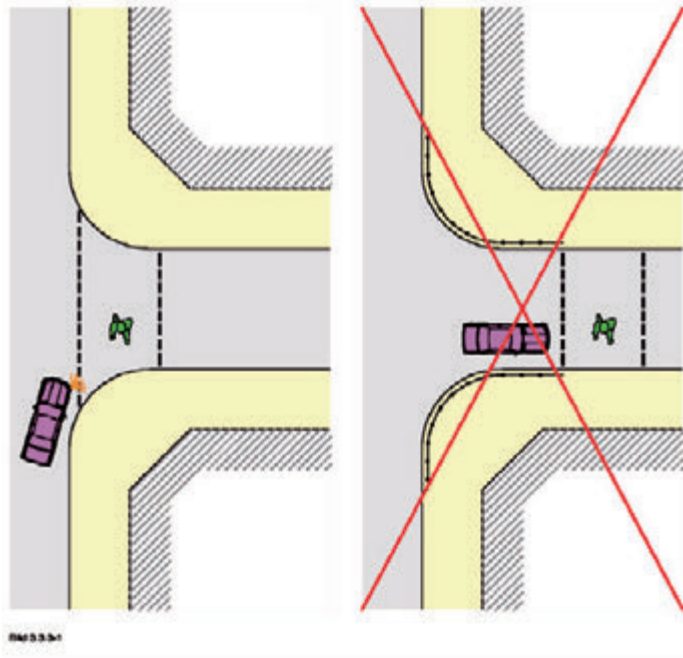
Abb. 15: links: nicht abgesetzte Querungsstelle (richtig), rechts: abgesetzte Querungsstelle (falsch), Quelle: H. Stadt (2012).
